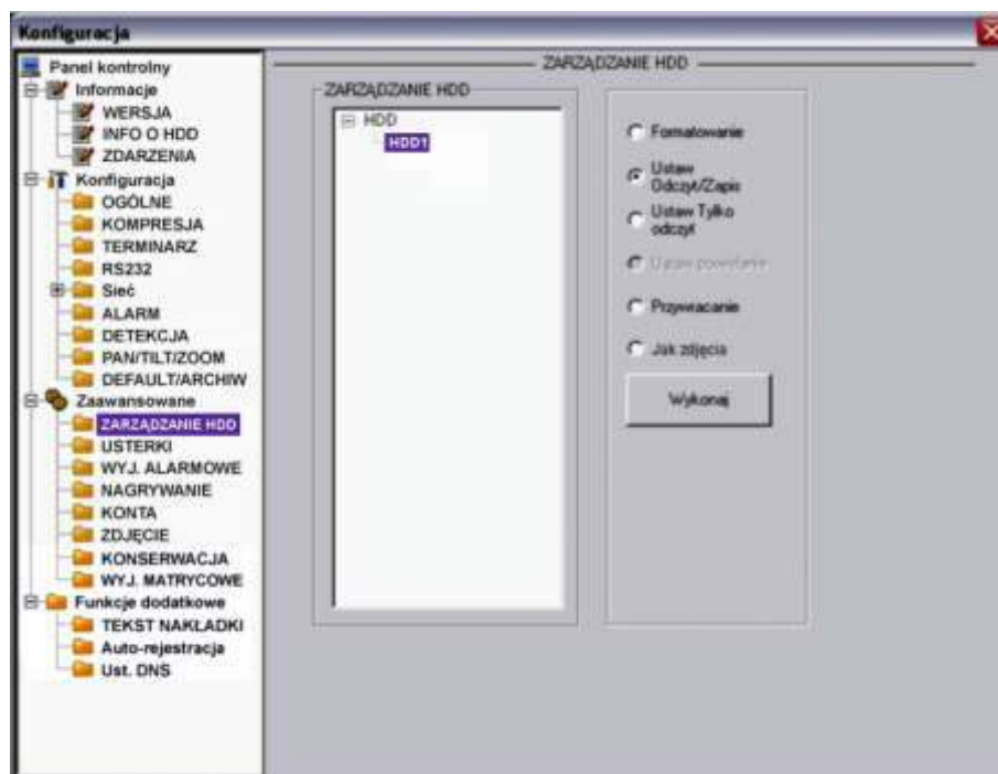
Rys. 7-46. Panel kontrolny → Zaawansowane → Zarządzanie HDD.
