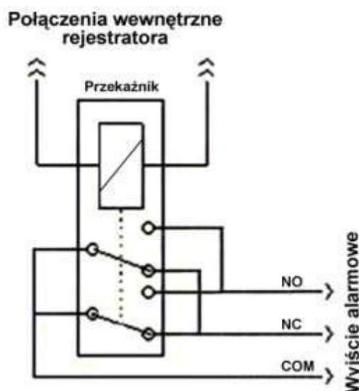
Rys. 3-9. Schemat wewnętrzny połączeń wyjścia alarmowego.
