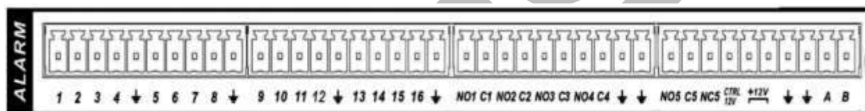
Rys. 3-6. Rozmieszczenia wejść / wyjść alarmowych rejestratora serii HE-T.
