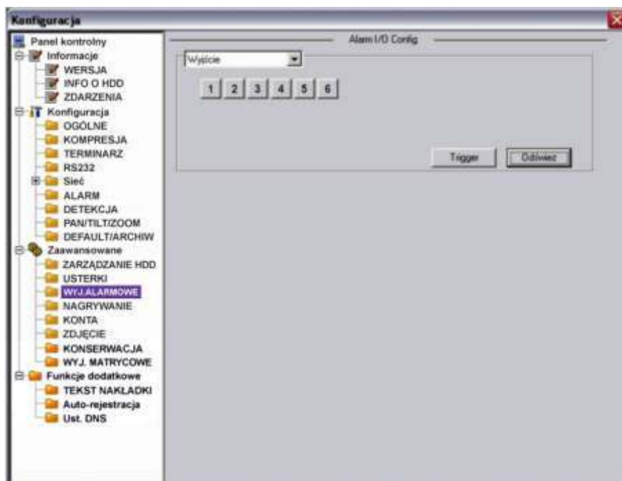
Rys. 7-48. Panel kontrolny → Zaawansowane → Alarm I/O Config.
