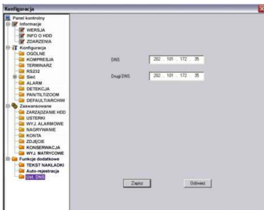
Rys. 7-56. Panel kontrolny → Funkcje dodatkowe → DNS.
