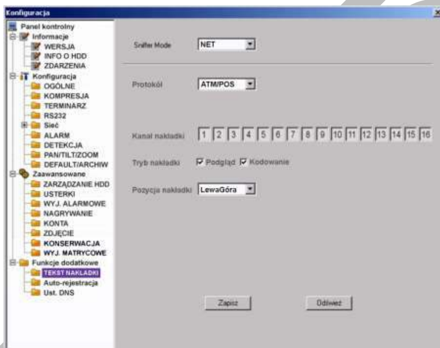
Rys. 7-54b. Panel kontrolny → Funkcje dodatkowe → Tekst nakładki – źródło NET.
