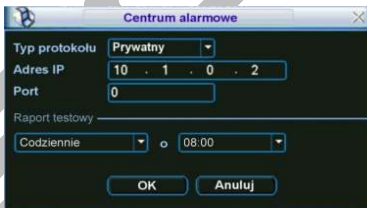
Rys. 5-17. Ustawianie serwera alarmowego.
