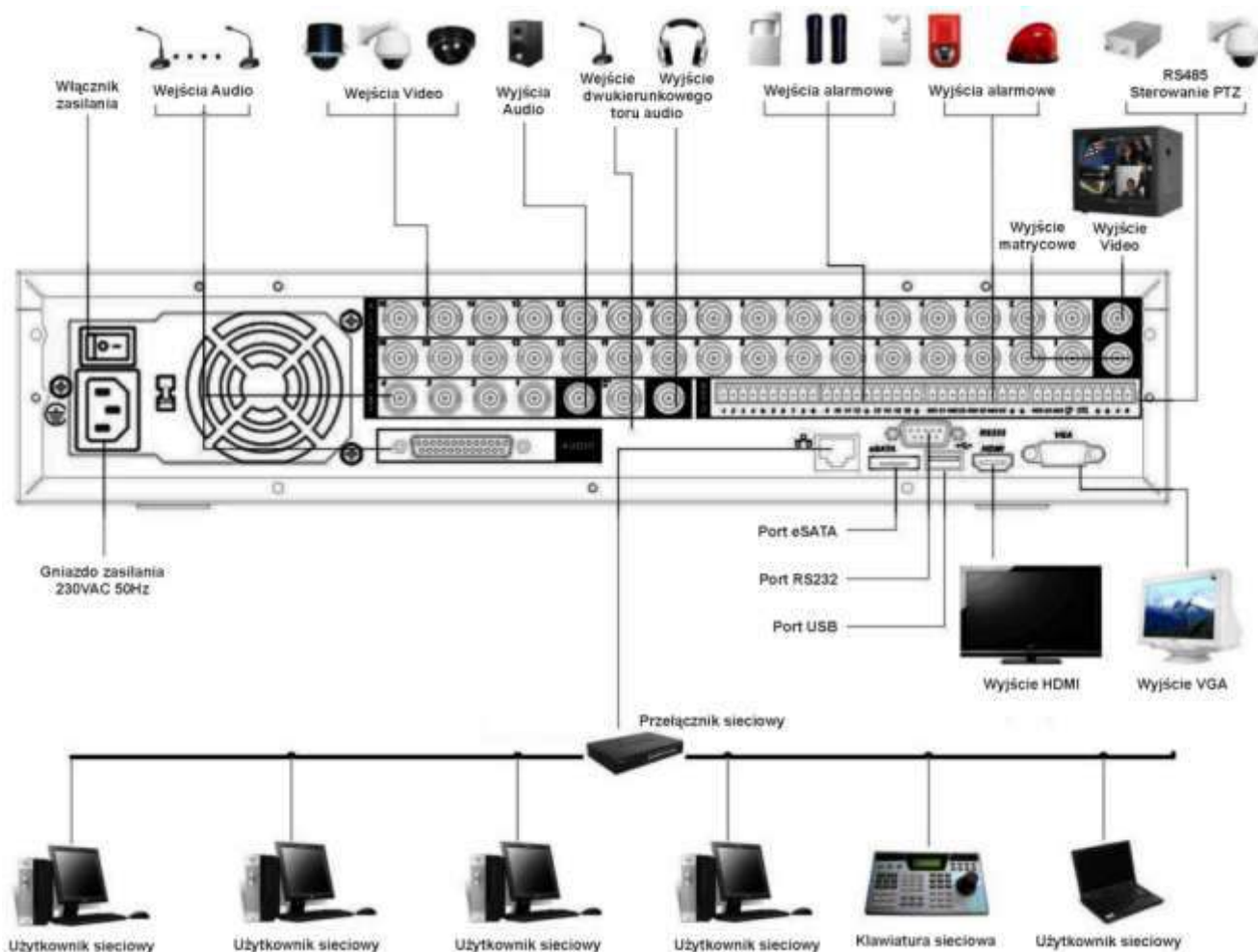
Rysunek 2-3. Przykładowy schemat podłączenia urządzeń peryferyjnych do rejestratora serii HE-T.
