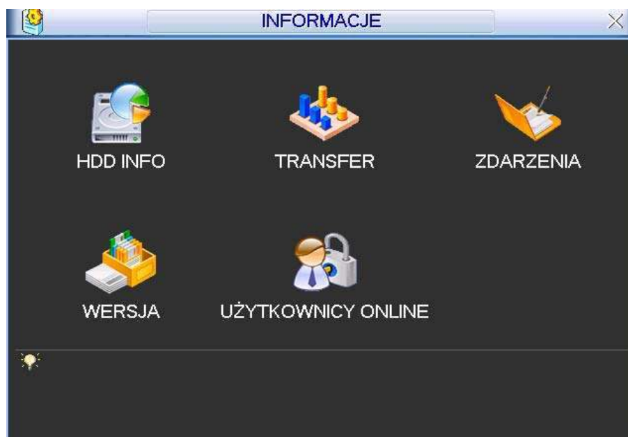
Rys. 5-40. Menu Informacje.
