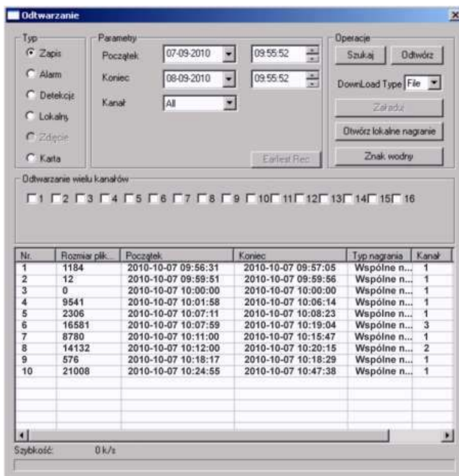
Rys. 7-58a. Interfejs Odtwarzanie.
