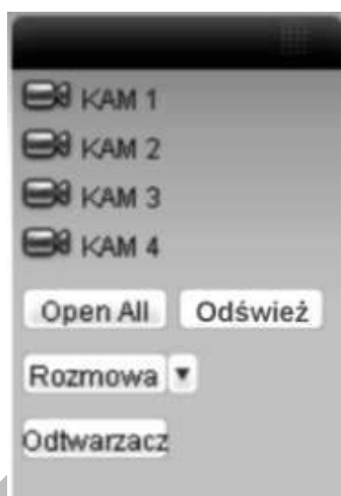
Rys. 7-5. Menu sekcji 2.
