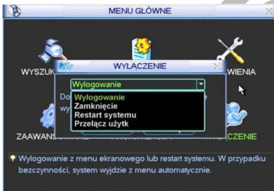
Rys. 5-47. Menu wyłączenie.
