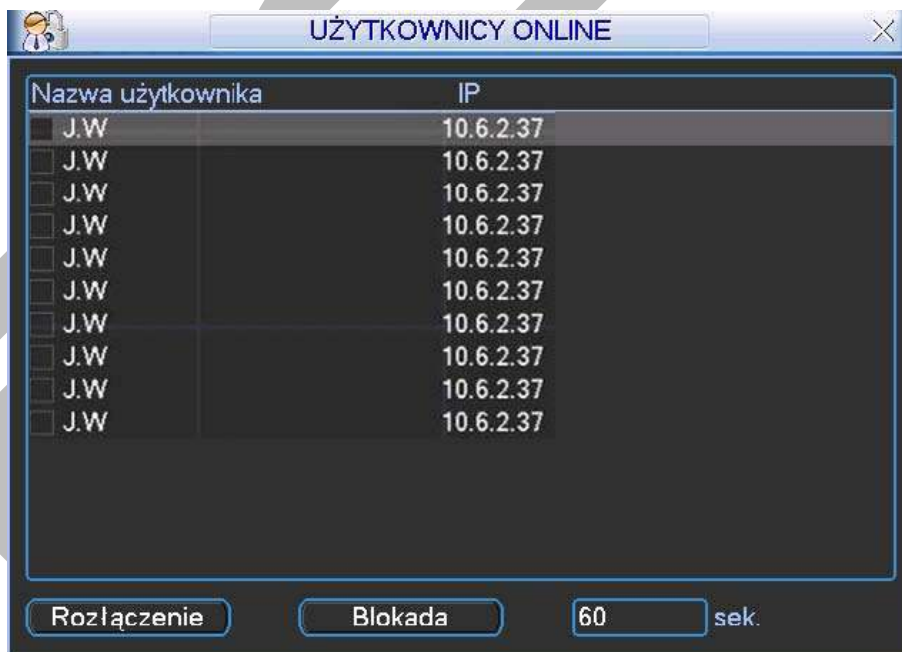
Rys. 5-46. Użytkownicy online.
