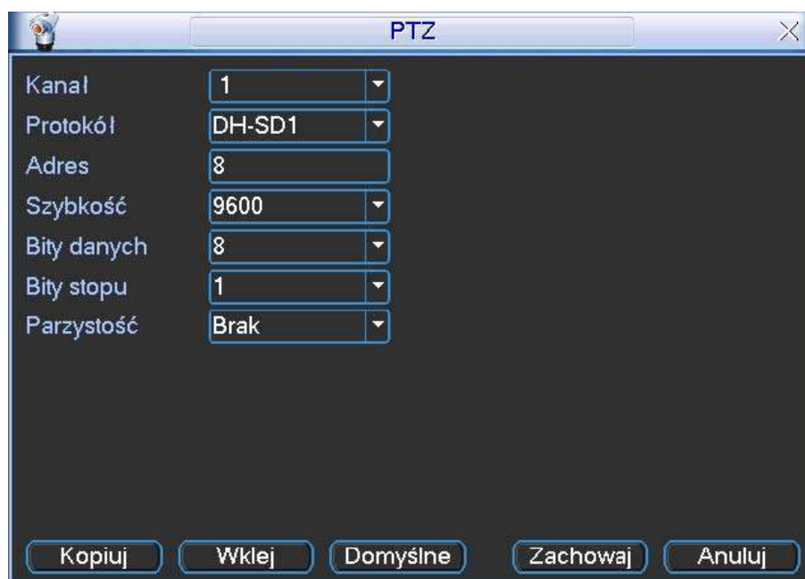
Rys. 4-29. Ustawienia PTZ.
