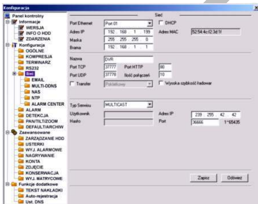
Rys. 7-34. Panel kontrolny → Konfiguracja → Sieć.
