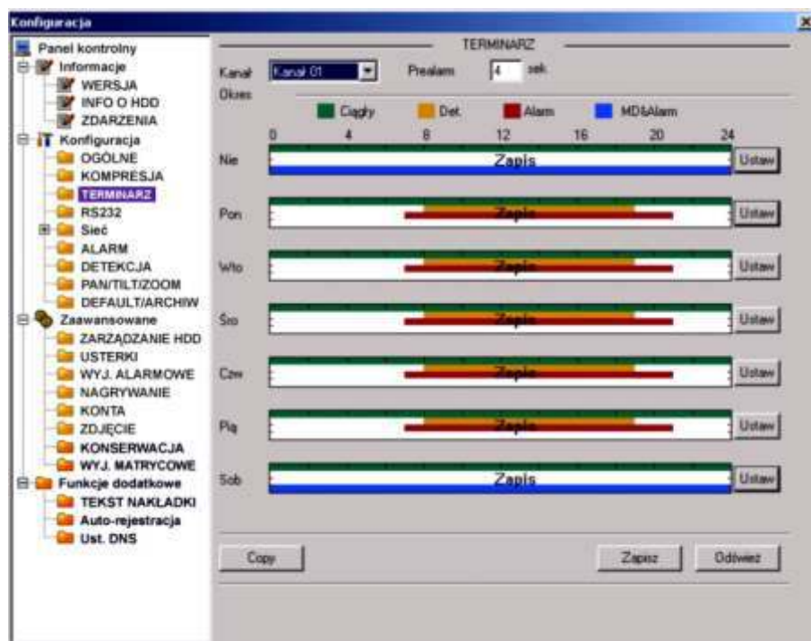
Rys. 7-30. Panel kontrolny → Konfiguracja → Terminarz.
