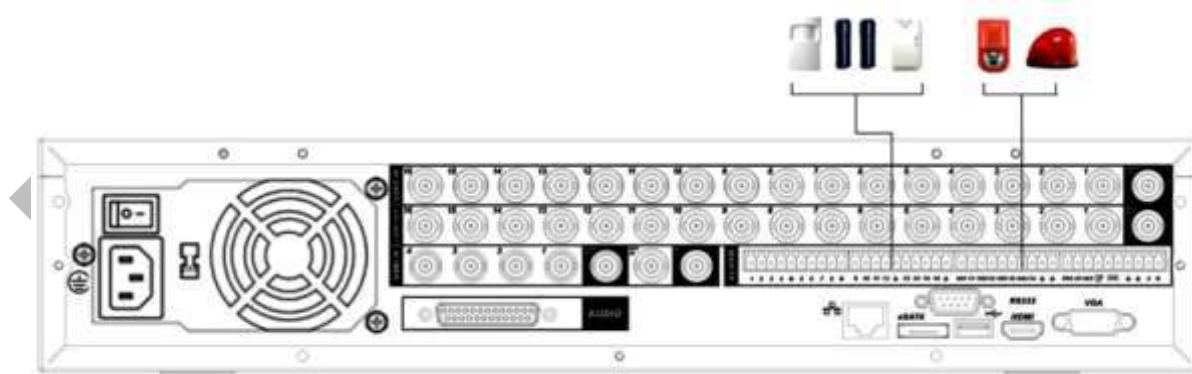
Rys. 3-5 Sposób podłączenia wejść i wyjść alarmowych.
