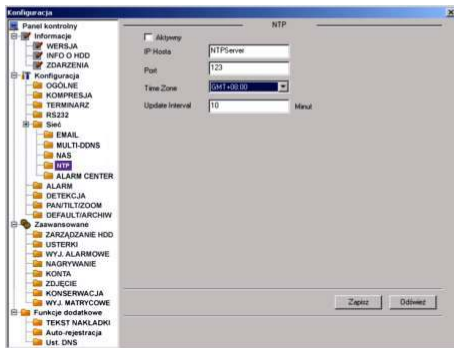
Rys. 7-37. Panel kontrolny → Konfiguracja → Sieć → NTP.
