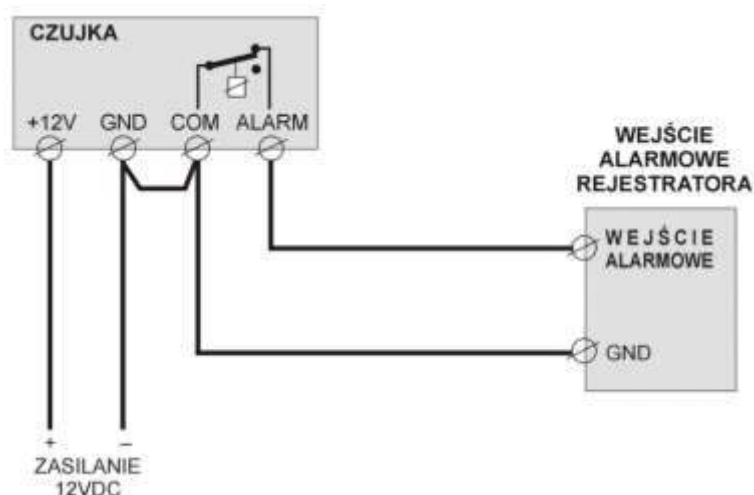
Rys. 3-7. Schemat podłączenia czujek do wejść alarmowych rejestratora.
