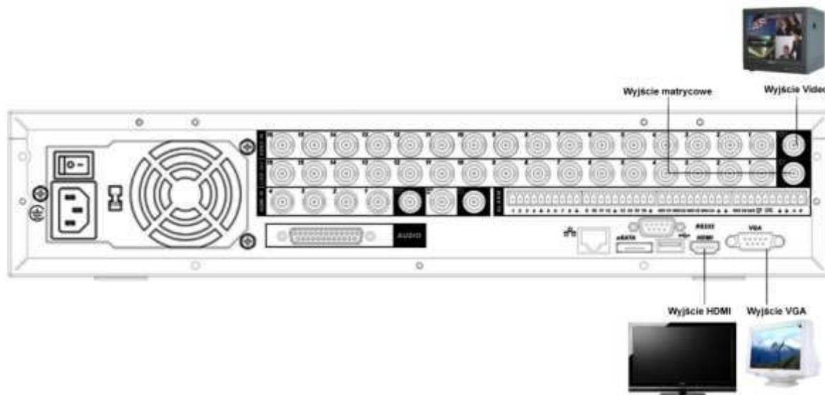
Rys. 3-4. Podłączenia do wyjść przelotowych i wyjścia matrycowego SPOT rejestratora.
