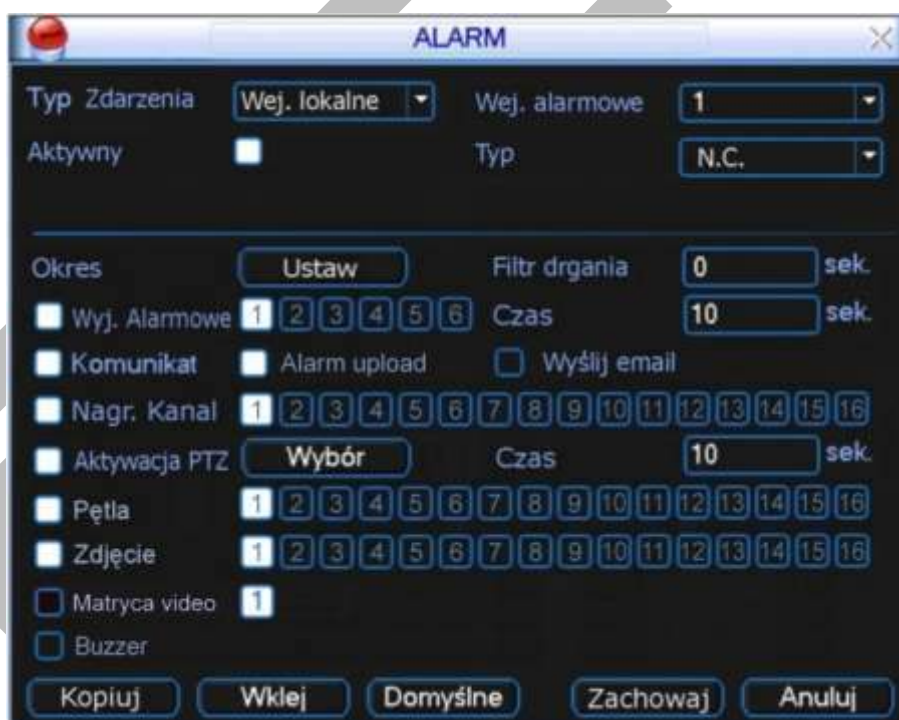
Rys. 4-15. Ustawianie parametrów zdjęcia w menu Alarm.
