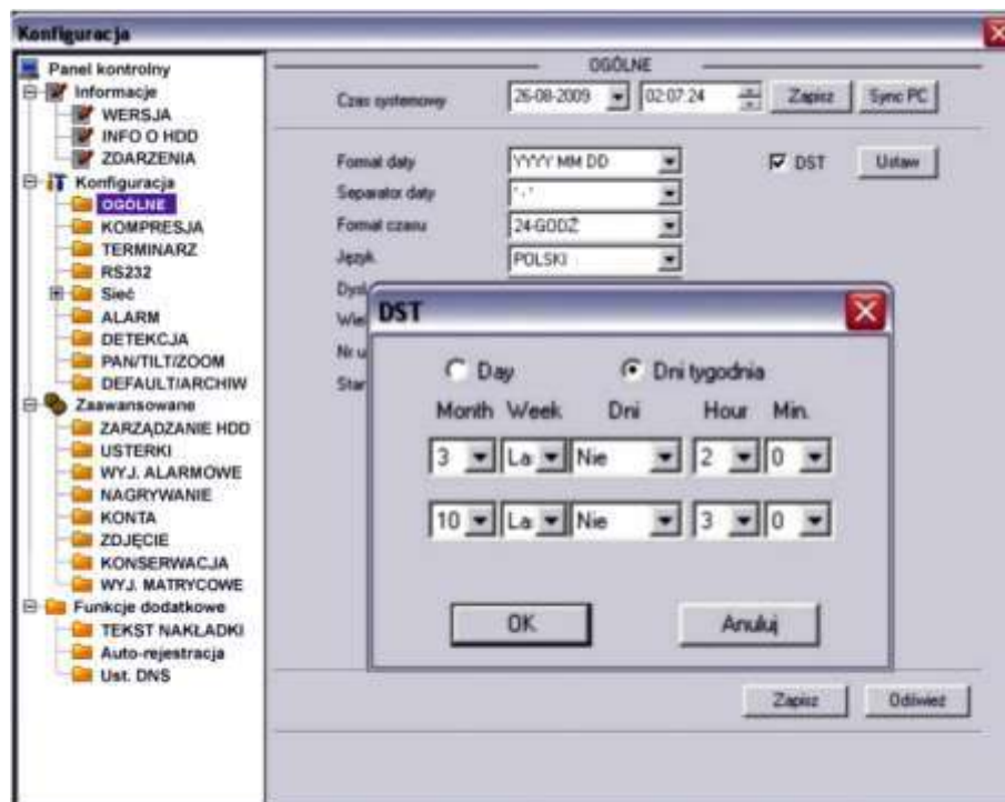
Rys. 7-27a. Ustawianie czasu letniego w menu Ogólne.
