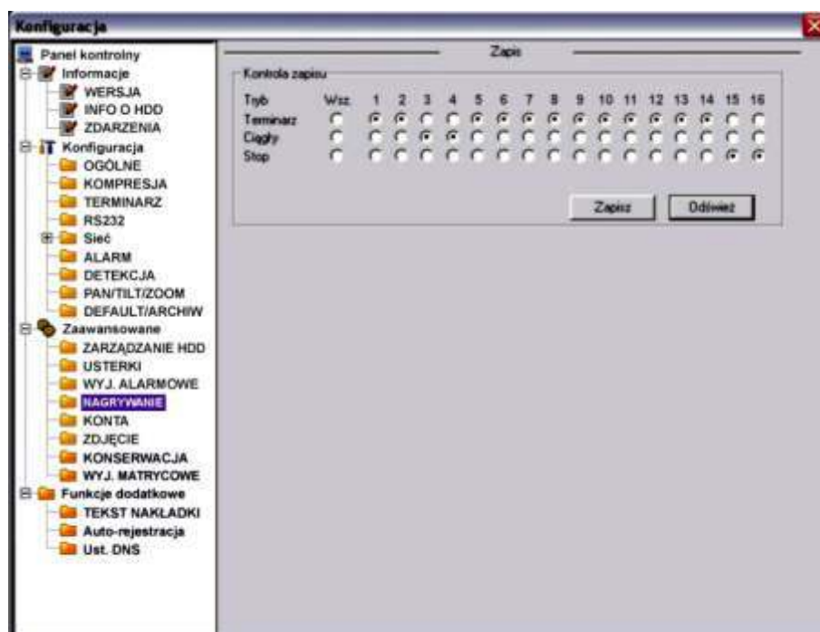
Rys. 7-49. Panel kontrolny → Zaawansowane → Zapis.
