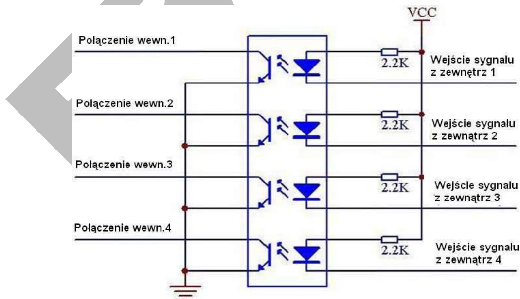
Rys. 3-8. Schemat wewnętrznych połączeń wejść alarmowych.
