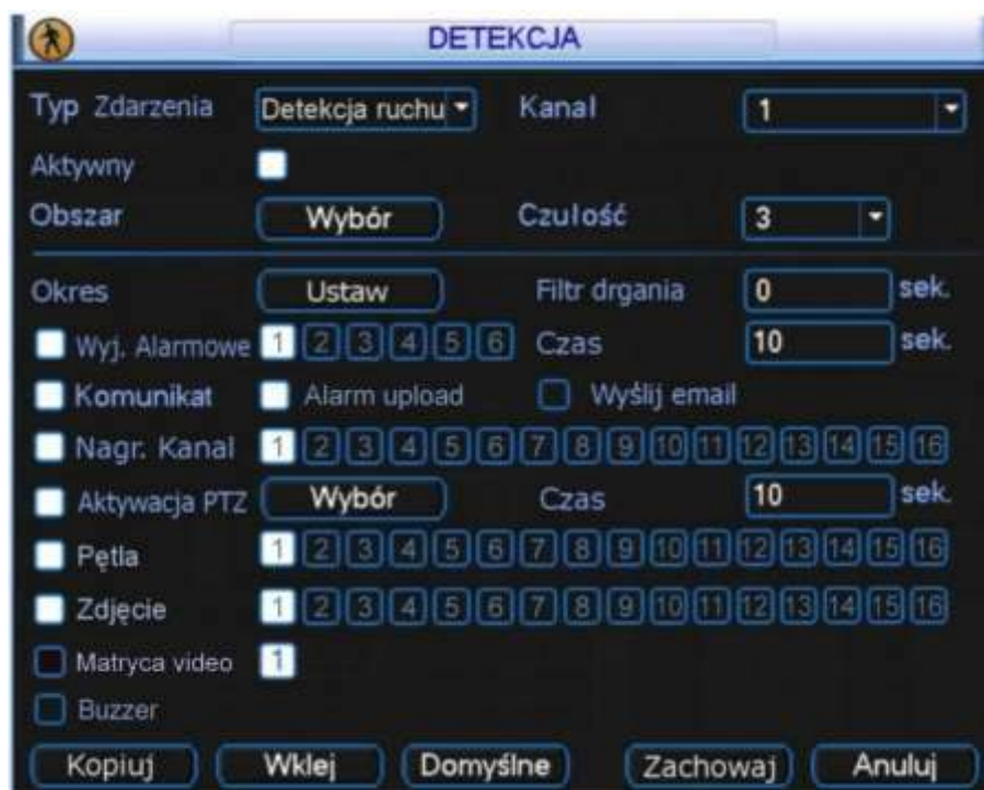
Rys. 4-17. Menu Detekcja.
