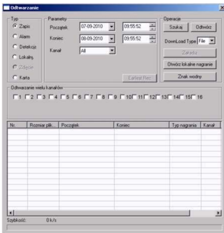
Rys. 7-58. Interfejs Wyszukiwanie.
